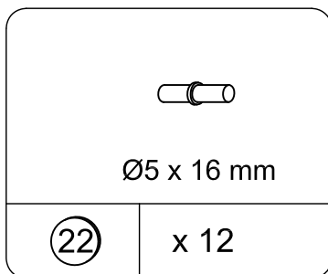
Shelf pin Pasador para el Tablero Taquet TWQ0018
