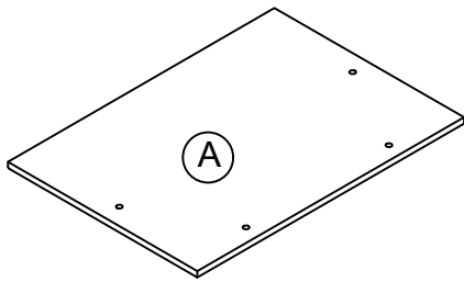
TOP TABLE T8969013010NN Qty: 1 PC
