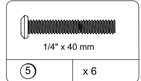
BOLT Perno BOULON TCS1064
