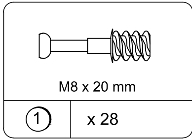
CAM BOLT Peron de la leva BOULON DE CAME TCS2010
