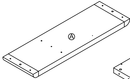
TOP Panel superior PANNEAU DESSUS T9548096010
