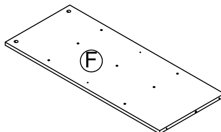
LEFT SIDE PANEL Panel lateral izquierdo PANNEAU GAUCHE T9654096061
